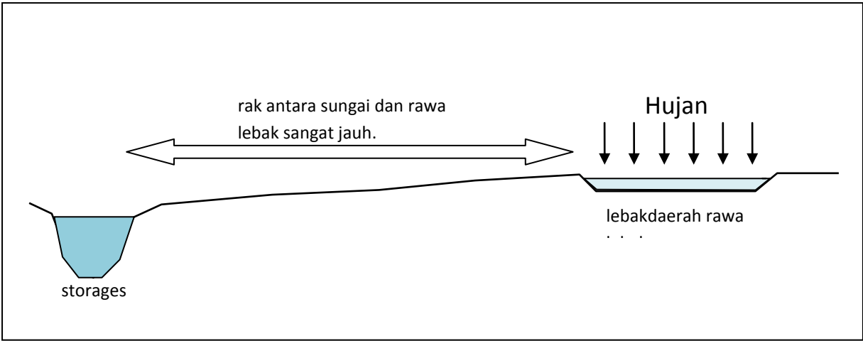
Gambar 6 Sistem tata air jaringan irigasi rawa lebak dengan tadah hujan.
