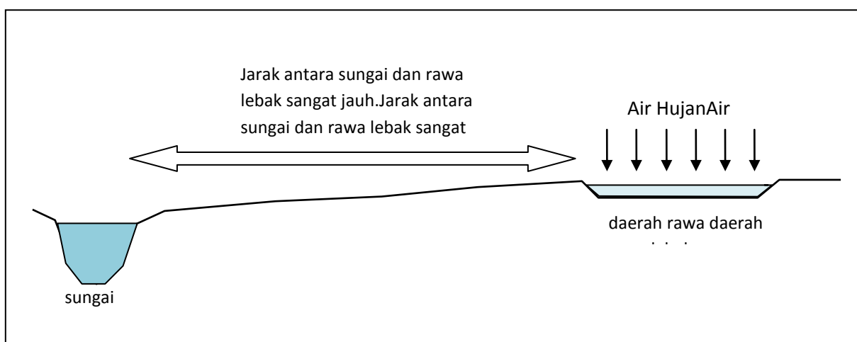
Gambar 2 Sistem tata air jaringan irigasi rawa lebak dengan tadah hujan.
