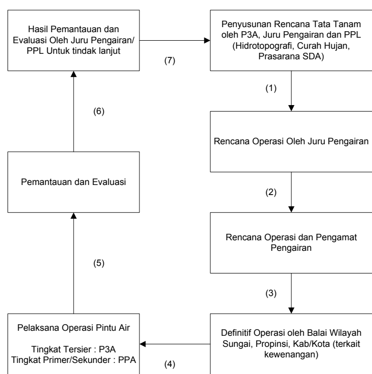
Gambar 5 Perencanaan operasi pintu air.
