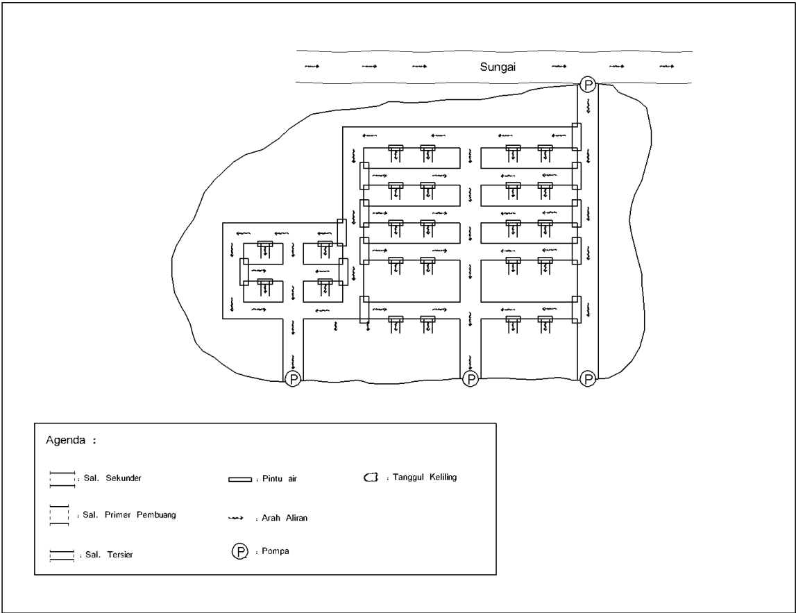
Gambar 14 Skema jaringan irigasi rawa lebak dengan sistem tata air polder Tipe pengairan ini dilakukan dengan cara memasang tanggul keliling yang dilengkapi dengan pompa untuk mengalirkan suplai air sungai ke daerah rawa (fungsi irigasi) ataupun sebaliknya (fungsi drainase). Tanggul keliling merupakan pematang besar yang berada di sekeliling sungai dan merupakan satu kesatuan dari sebuah sistem polder yang berfungsi mengurangi limpahan air sungai pada musim hujan dan pada muara saluran utama didirikan pintu pengendali banjir. Penggunaan pompa digunakan agar pada musim kemarau suplai air dari sungai bisa tetap dialirkan ke daerah rawa. Sistem Tata air dari jaringan irigasi rawa lebak yang menggunakan sistem tata air tanggul (polder) dapat dilihat pada Gambar 15 .
